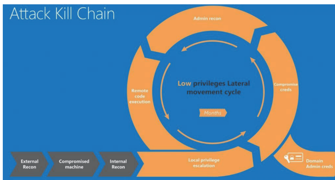
图 2.3.4 Kill Chain 模型攻击过程
